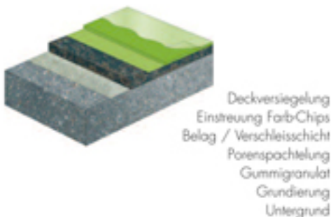
Bodenaufbau Durapur Comfortbelag Flexitan Schichtstärke 8-12mm 18-22Db
