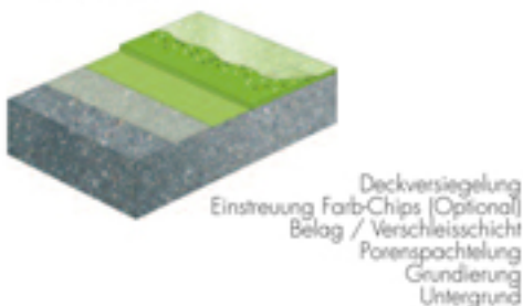
Bodenaufbau Durapur Fließbelag Schichtstärke 2-3mm
