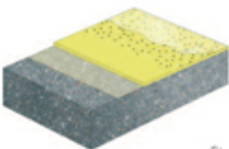
Bodenaufbau Duracon Color-Vollchipsbelag Schichtstärke 2-3mm
