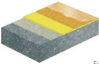
Bodenaufbau Duracon Colorquarzbelag Schichtstärke 2-3mm
