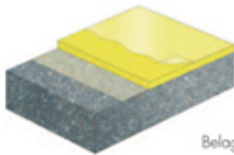
Bodenaufbau Duracon Mörtelbelag Schichtstärke 5-8mm
