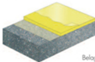
Bodenaufbau Duracon Mörtelbelag Schichtstärke 5-8mm
