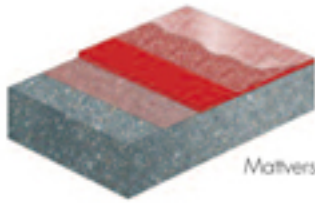
Bodenaufbau Durapox Colorquarzbelag Schichtstärke 2-3mm
