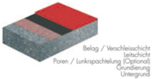
Bodenaufbau Durapox AS-Belag Schichtstärke 2-3mm
